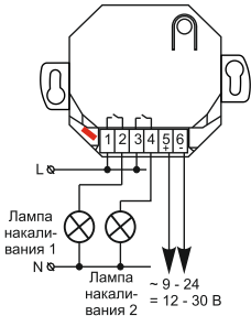
Рисунок 2. Схема подключения к двум лампам накаливания
