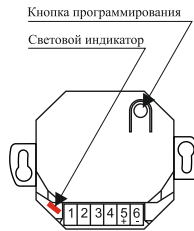
Рисунок 4. Расположение элементов управления и индикации
